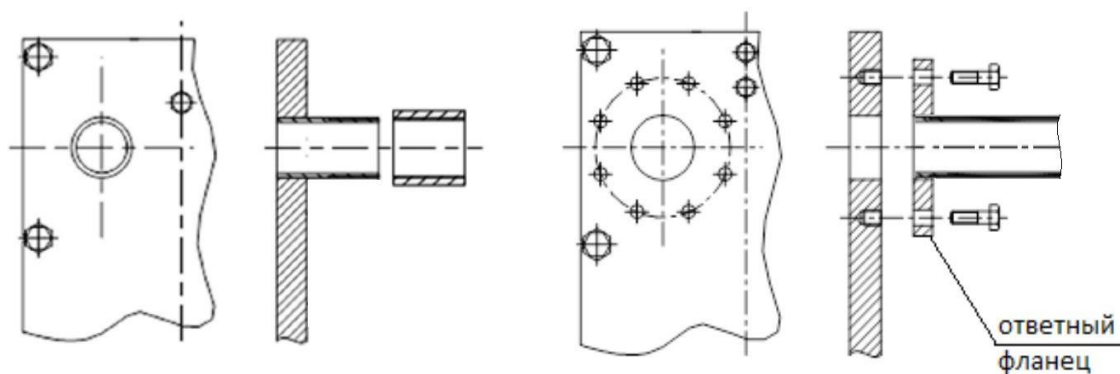
Рисунок А.2 – Схема подключения трубопроводов к теплообменнику
