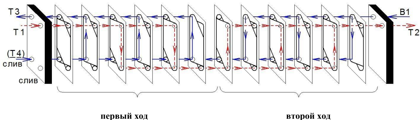
Рисунок 4- Компоновка пластин двухходового теплообменника (с циркуляционной линией Ц)
