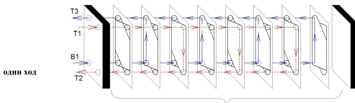
Рисунок 2- Компоновка пластин одноходового теплообменника с расположением патрубков на неподвижной плите
