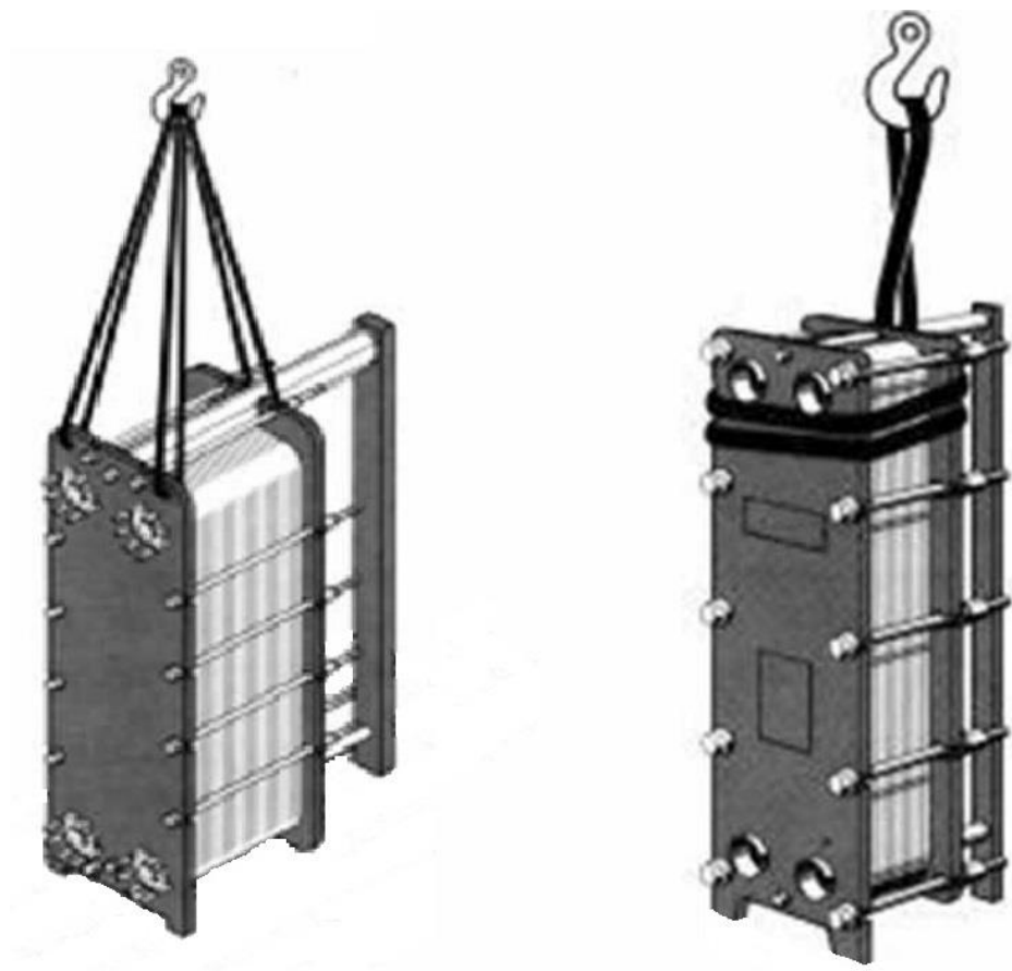
Рисунок А.1 – Схема строповки теплообменника
