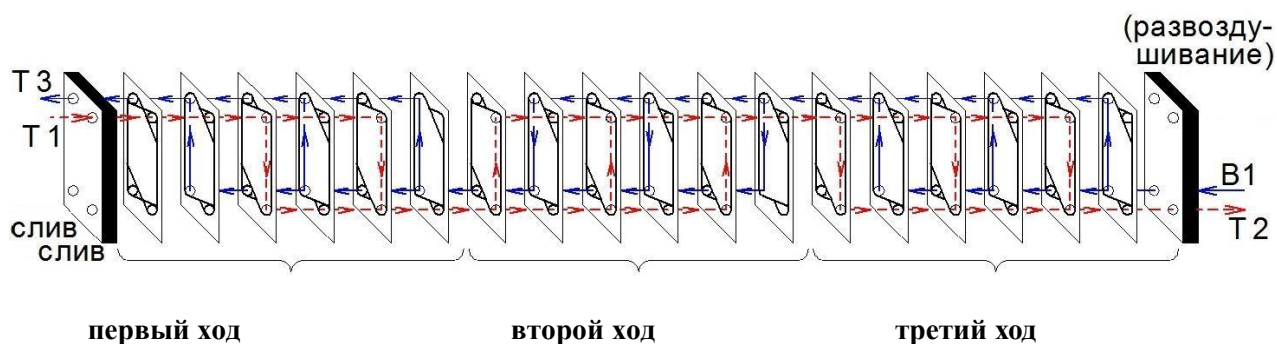
Рисунок 6- Компоновка пластин трехходового теплообменника
