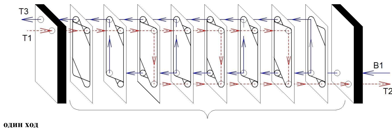
Рисунок 3- Компоновка пластин одноходового теплообменника с расположением патрубков с разных сторон теплообменника
